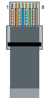
EIA/TIA 568B
